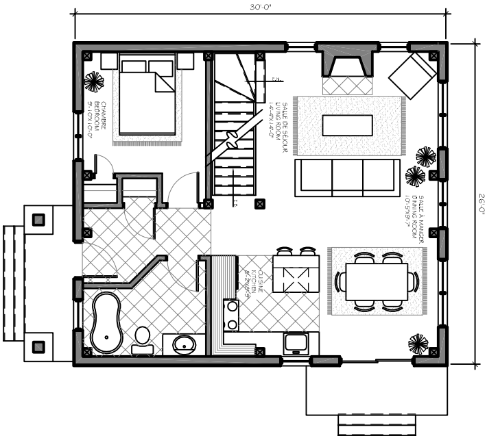
PLAN DU REZ-DE-CHAUSSÉE GROUND FLOOR PLAN 780 p.l.ca. / sq.ft.
