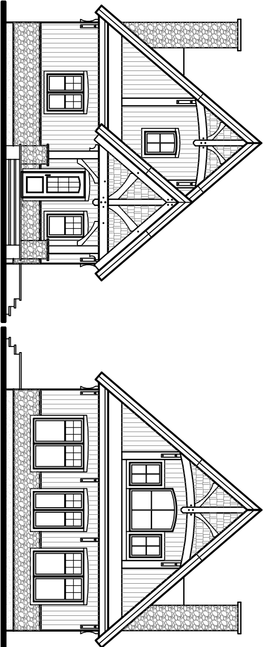
ÉLÉVATION AVANT FRONT ELEVATION
