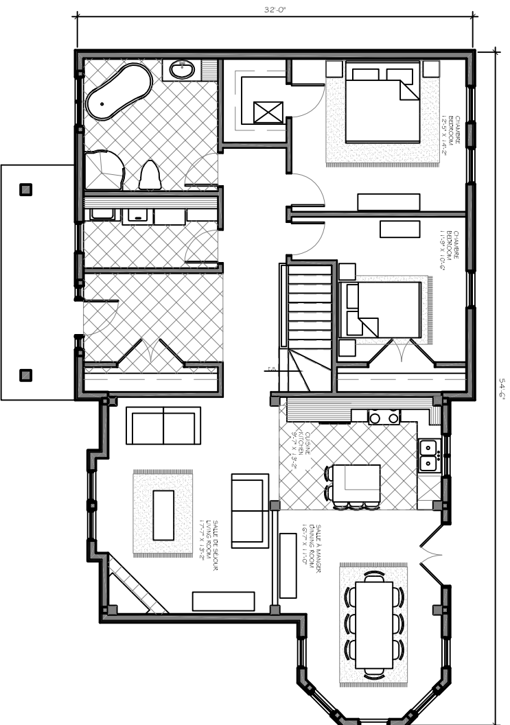
PLAN DU REZ-DE-CHAUSSÉE GROUND FLOOR PLAN 1 496 p.i.ca. / sq.ft.
